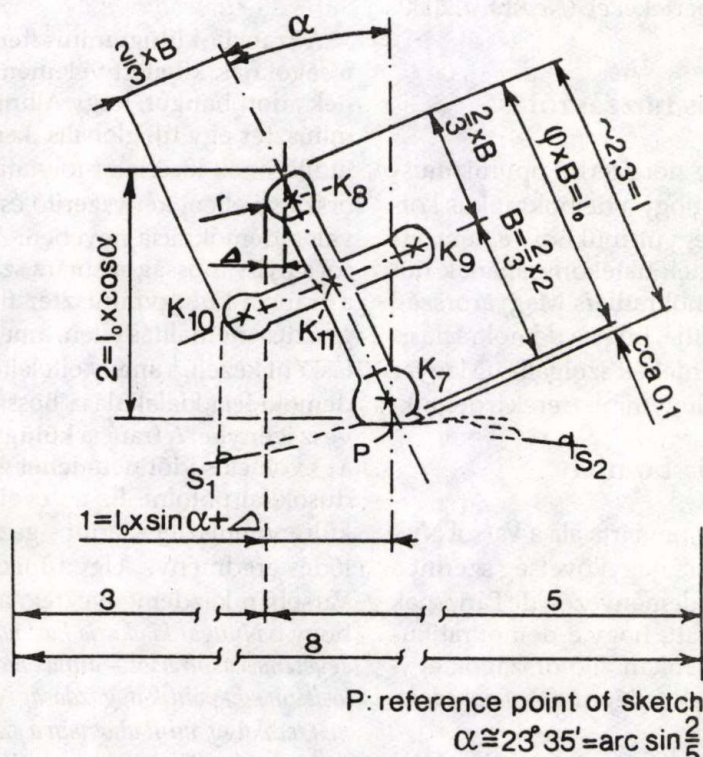
A ferde kereszt rajza. Méretek és dőlési szög. Cikket lásd a 35. oldalon
